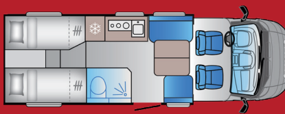
C 70 DL 699 cm Ford Eco Blue 165 PS Euro 6 mit Automatik ab € 59.990,- *
